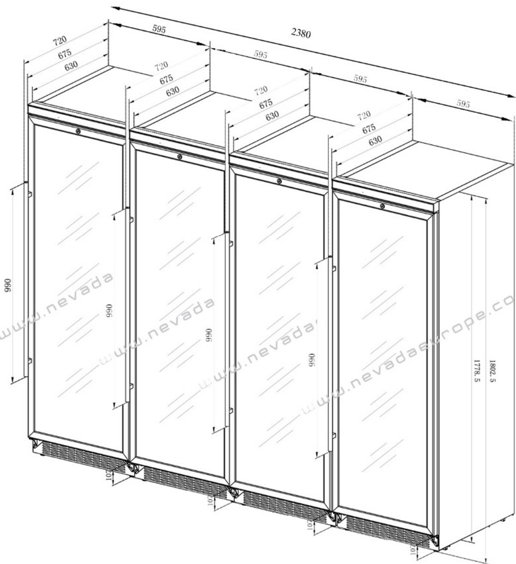
Dimensioni Cantina Nevada NW518Q2-SL
